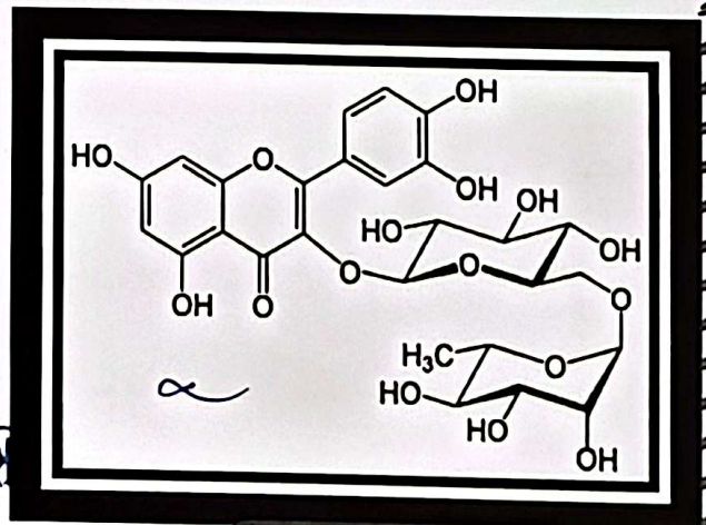
Rutin
