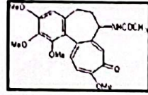
Colchicine
